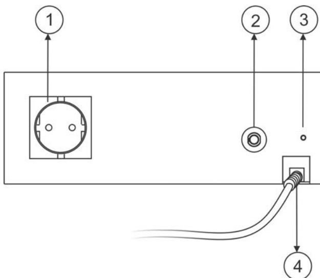
شکل ۲: پنل پشت
